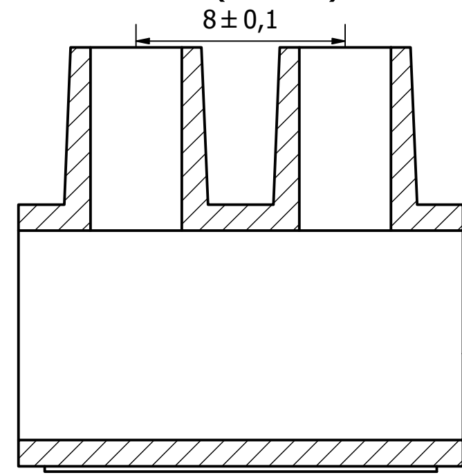
A-A ( 5 : 1 )
